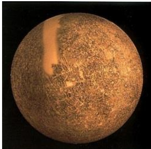
Orbita Merkurego
